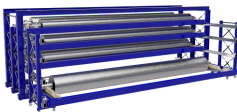
Bloc tiroir pour rouleaux de 10 m 12 t par extension transversale
